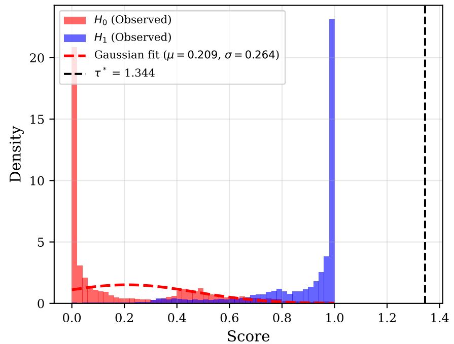
CNN-2feat
