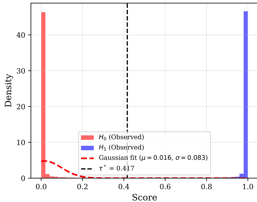
SVM
